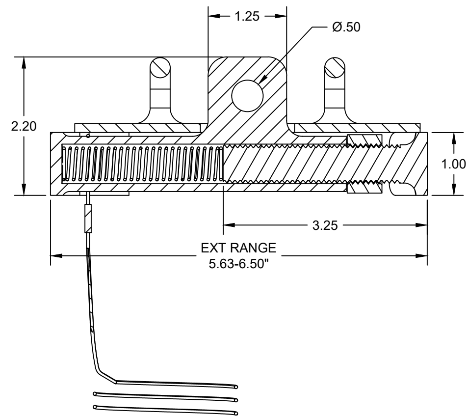
SECTION A-A
